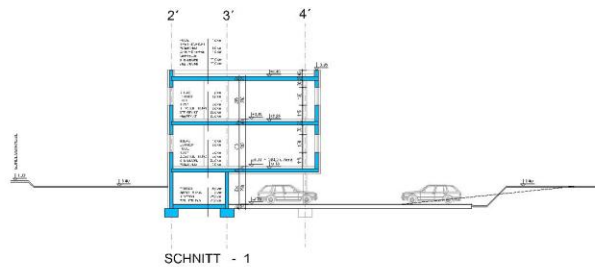
SCHNITT - 1
